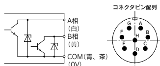
ものさしくんの出力回路
