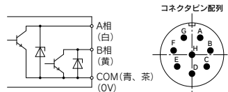
ものさしくんの出力回路
